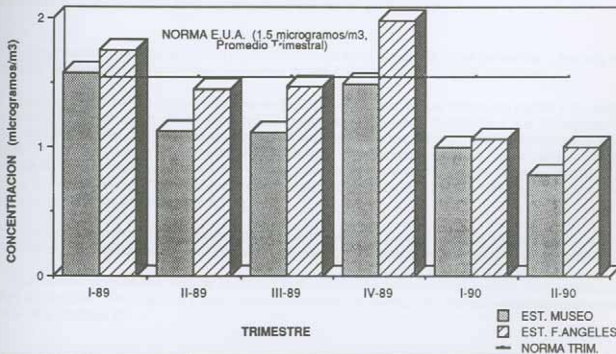
GRAFICA 8. PROMEDIOS TRIMESTRALES DE PLOMO DURANTE 1989 Y PRIMER SEMESTRE DE 1990
