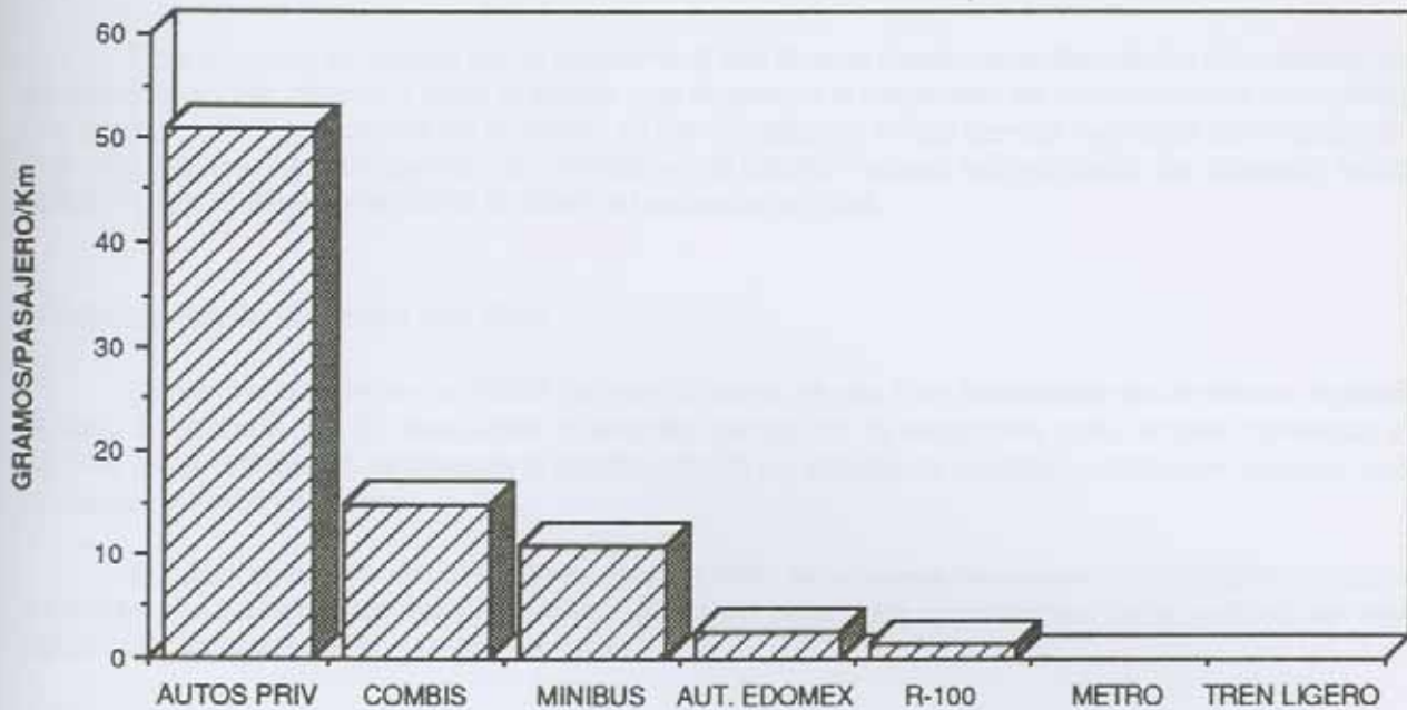
GRAFICA 17. EMISION DE CONTAMINANTES POR MODO DE TRANSPORTE
