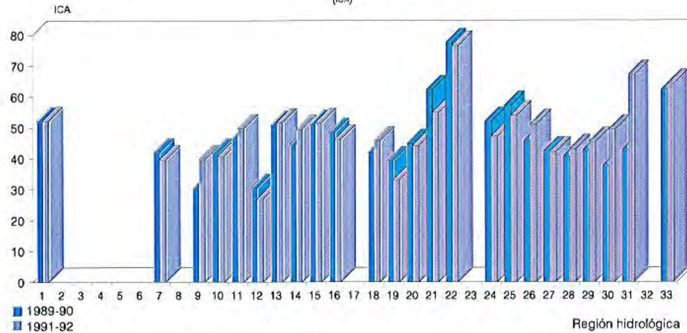
Gráfica 12 Índice de la calidad del agua (ICA)
