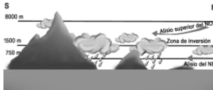
Fig. 22. Esquematación del efecto orográfico
